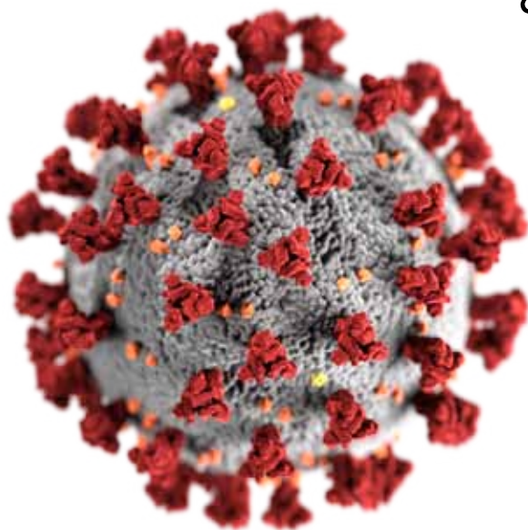
Wizualizacja wirusa SARS-CoV-2
